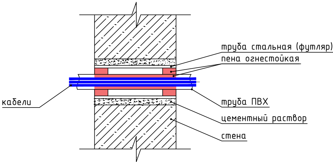
Узел прохода кабельной линии через стену, перекрытие
